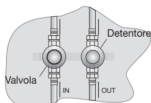
Allacciamento del GVR all'impianto Idraulico
