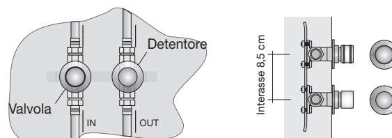
Allacciamento del GVR all'impianto Idraulico
