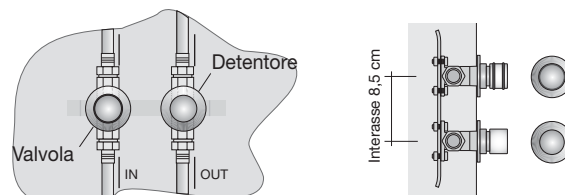
Allacciamento del GVR all'impianto Idraulico
