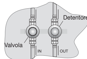
Allacciamento del GVR all'impianto Idraulico
