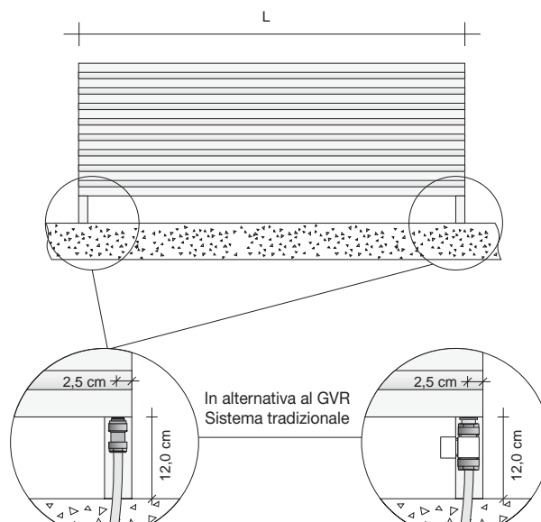
Allacciamento al GVR Gruppo Valvole Remoto Attacchi SH1
